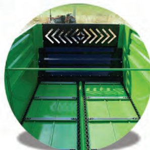
Sistema transportador de cadena de doble fila Sistema transportador de corrente de duas fileiras
