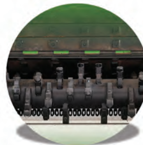
Rotor trituradora de metal duro Rotor de britador de carboneto
